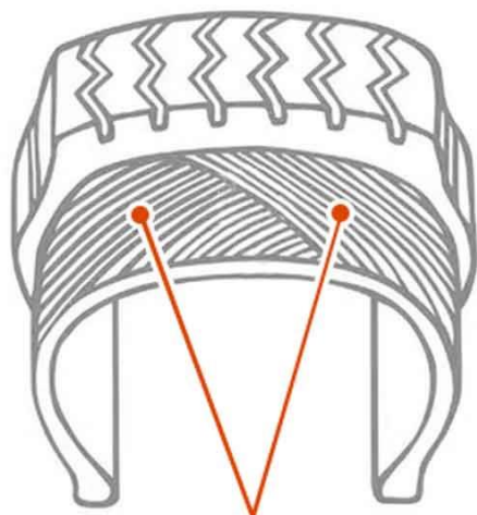
لاستیک بایاس
