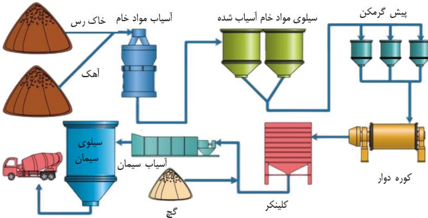
شکل ۲- فرآیند تولید سیمان
