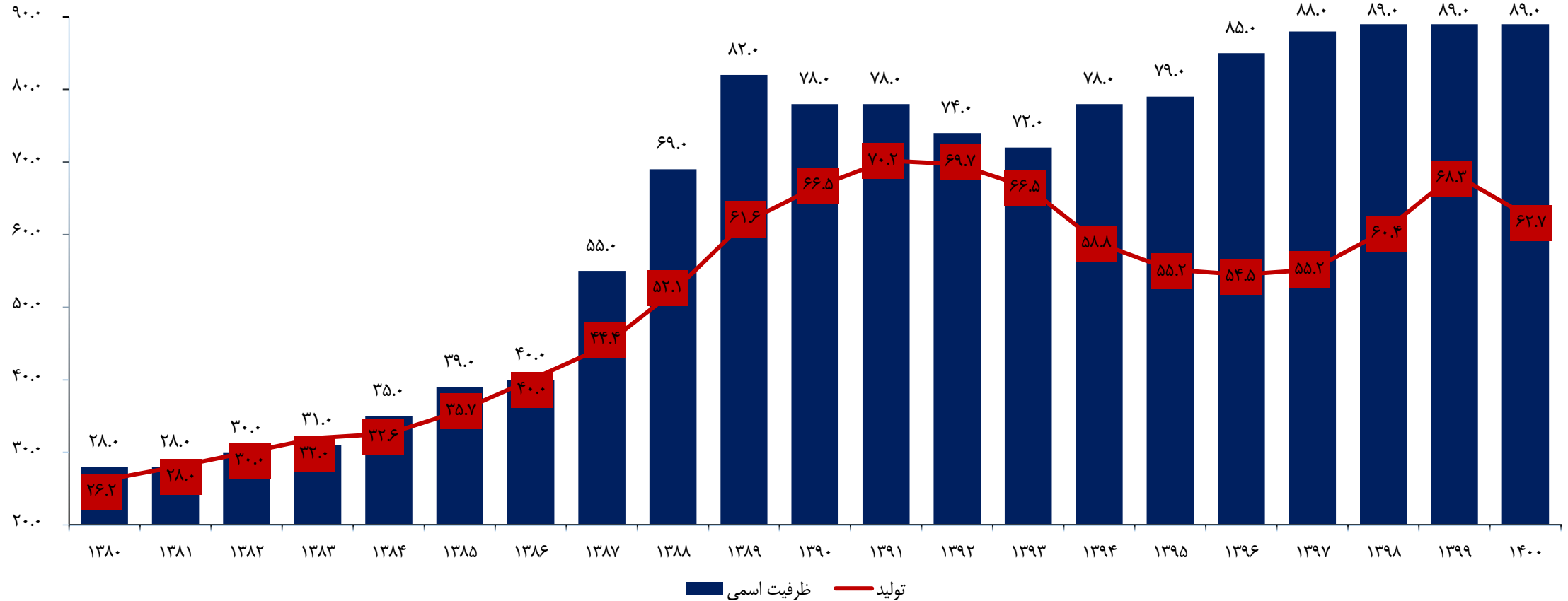
نمودار ۶- ظرفیت اسمی و تولید سیمان کشور (میلیون تن)
