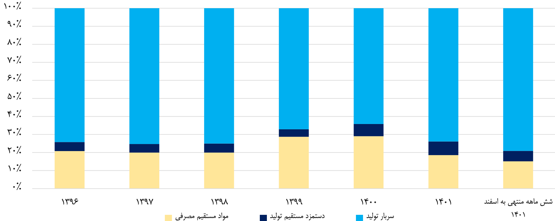
نمودار ۱۳- اجزای تشکیل دهنده بهای تمام شده (درصد)
