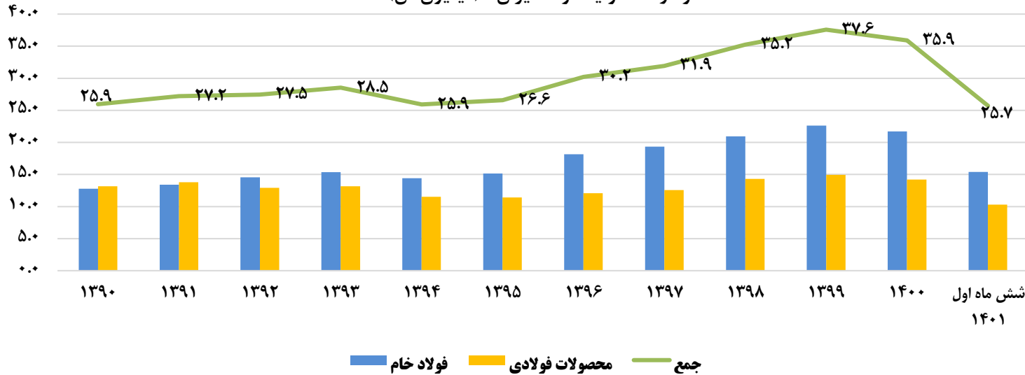
نمودار ۱۵- تولید فولاد ایران - (میلیون تن)
