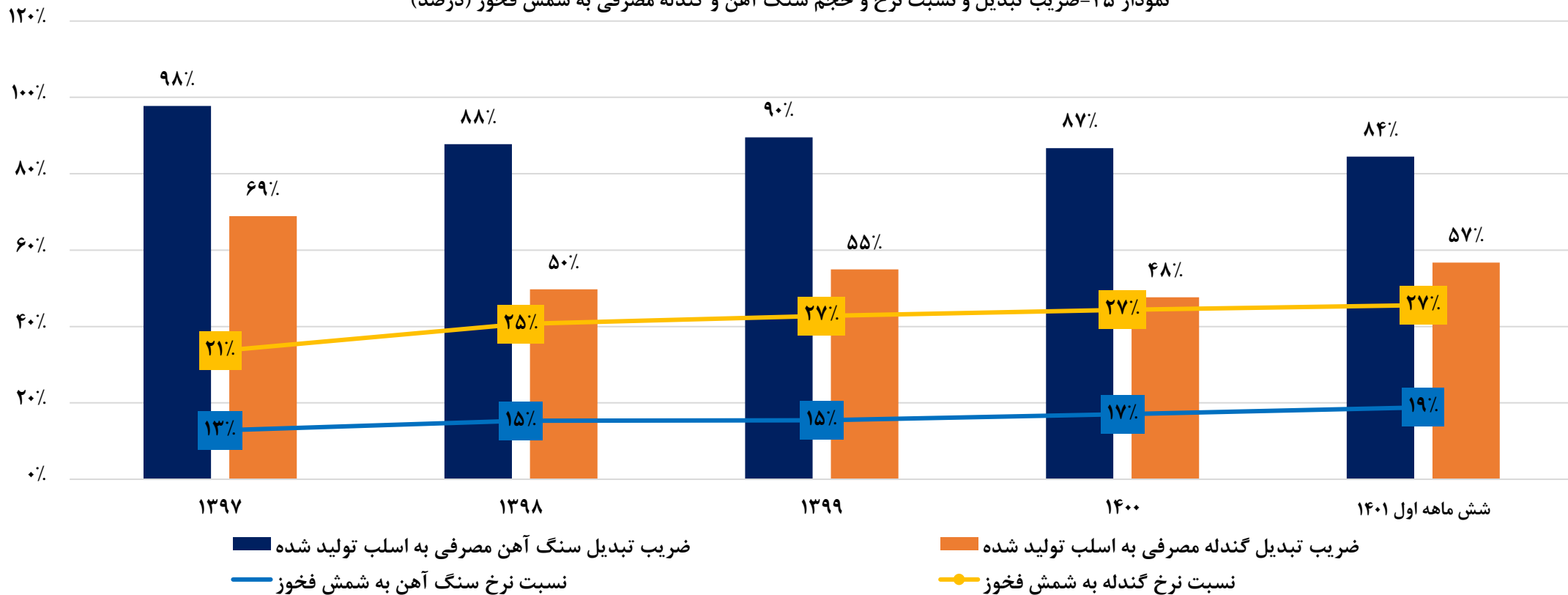
نمودار ۲۵- ضریب تبدیل و نسبت نرخ و حجم سنگ آهن و گندله مصرفی به شمش فخوز (درصد)
