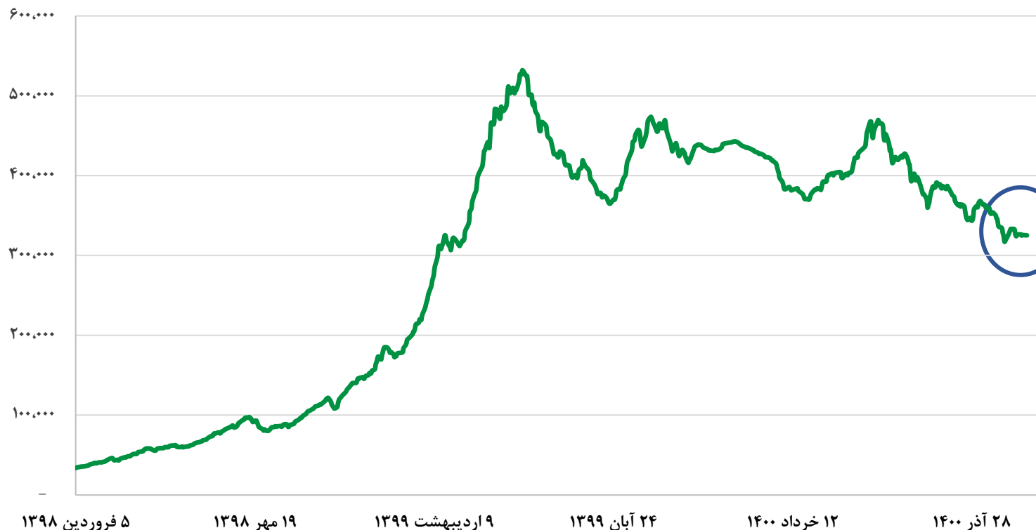
نمودار شاخص هم وزن از ابتدای ۱۳۹۸
